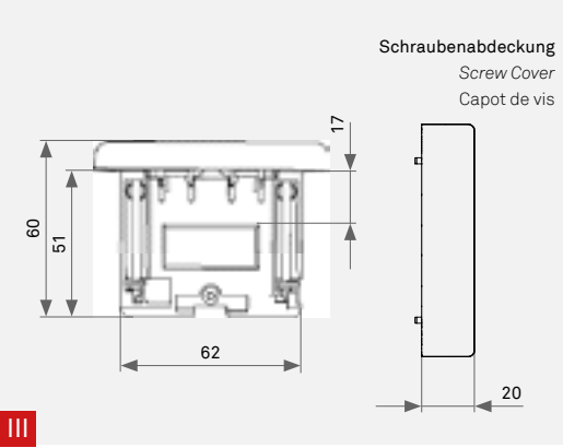
Maße | Dimensions | Dimensions mm FrameDock Hide
