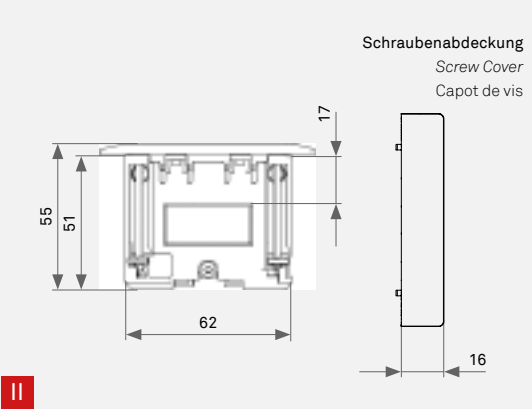
Maße | Dimensions | Dimensions mm FrameDock
