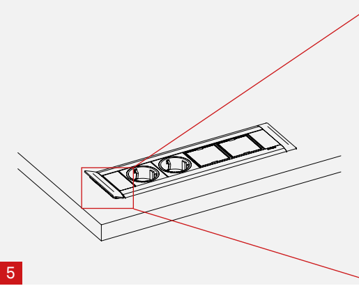
Einbauanleitung | Installation Instructions | Guide d'installation FrameDock Hide
