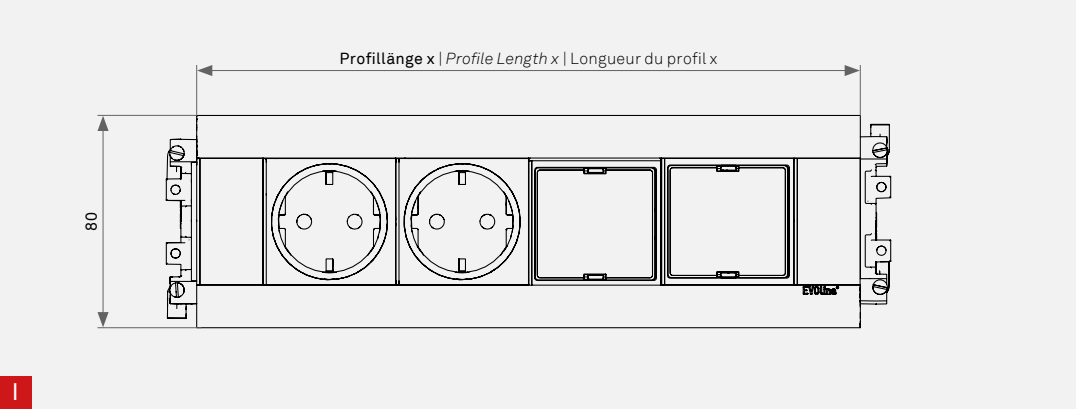
Maße Tischausschnitt | Dimensions Table Cutout | Dimensions de la découpe mm FrameDock & FrameDock Hide
