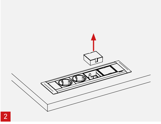
Austausch Wechselmodul | Replacement of an interchangeable module | Remplacement d'un module interchangeable FrameDock & FrameDock Hide
